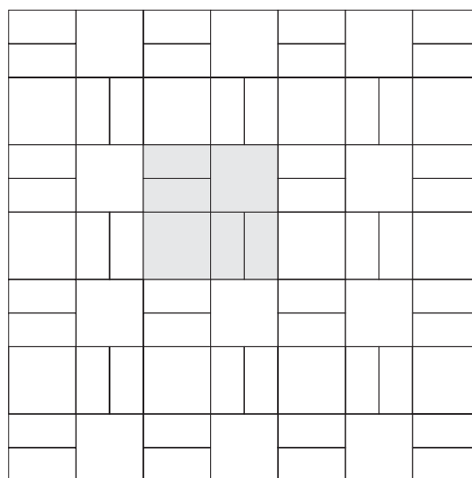
D 9,8 x 19,8 cm env. 25 pièces/m 2 / ca. 25 St./m 2 19,8 x 19,8 cm env. 12,5 pièces/m 2 / ca. 12,5 St./m 2
