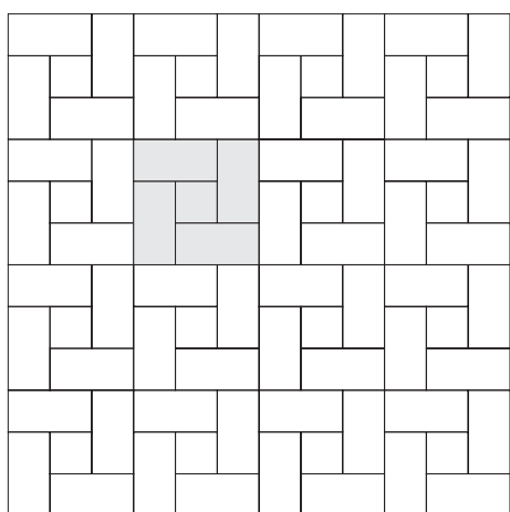
C 9,8 x 9,8 cm env. 11 pièces/m 2 / ca. 11 St./m 2 9,8 x 19,8 cm env. 44,5 pièces/m 2 / ca. 44,5 St./m 2
