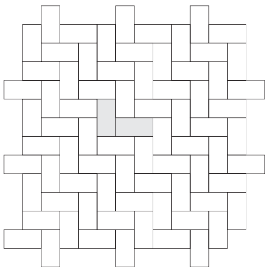
A 9,8 x 19,8 cm env. 50 pièces/m 2 / ca. 50 St./m 2
