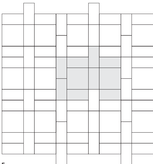
E 9,8 x 19,8 cm env. 29 pièces/m 2 / ca. 29 St./m 2 19,8 x 19,8 cm env. 10,5 pièces/m 2 / ca. 10,5 St./m 2
