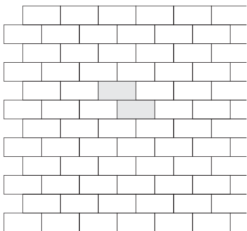
A 19,8 x 9,8 cm env. 50 pièces/m 2 / ca. 50 St./m 2
