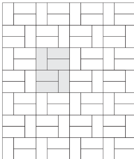
D 19,8 x 9,8 cm env. 50 pièces/m 2 / ca. 50 St./m 2
