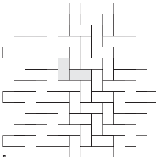
B 19,8 x 9,8 cm env. 50 pièces/m 2 / ca. 50 St./m 2
