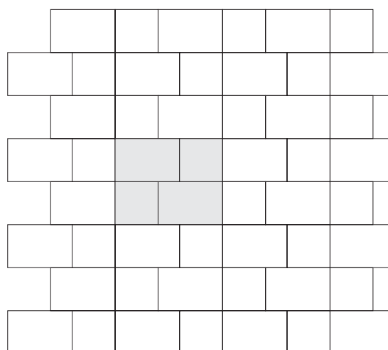
D 15,8 x 15,8 cm env. 16 pièces/m 2 / ca. 16 St./m 2 23,8 x 15,8 cm env. 16 pièces/m 2 / ca. 16 St./m 2
