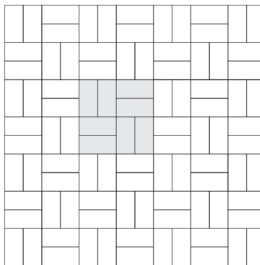
D 9,8 x 19,8 cm env. 50 pièces/m 2 / ca. 50 St./m 2
