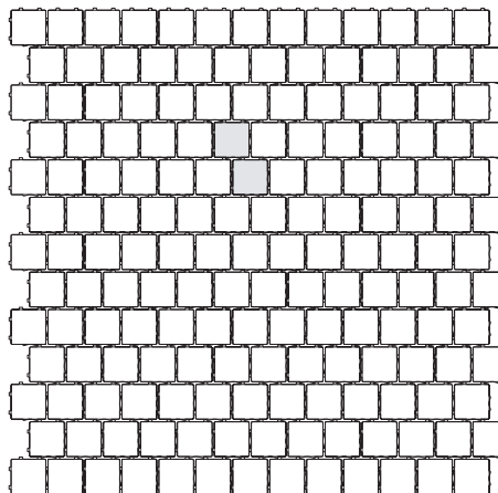
B Joints drainants / Drainfügen 18,5 x 18,5 cm env. 29 pièces/m 2 / ca. 29 St./m 2
