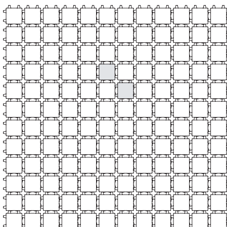
C Joints engazonnés / Rasenfügen 20 x 20 cm env. 25 pièces/m 2 / ca. 25 St./m 2
